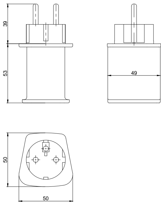
Габаритные размеры
